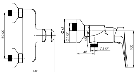
DELI-12 Shower faucet | D20008
