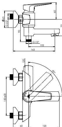
DELI-10 (SW) (K) Vaňová / sprchová batéria so sprchovým setom | D1PK08
