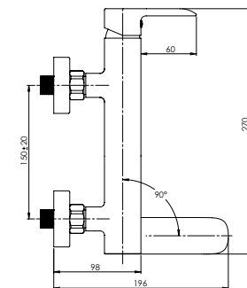
ULTRA-10 (SW) (K) Vaňová / sprchová batéria so sprchovým setom | U1KP08 | LUX: U1KPL08
