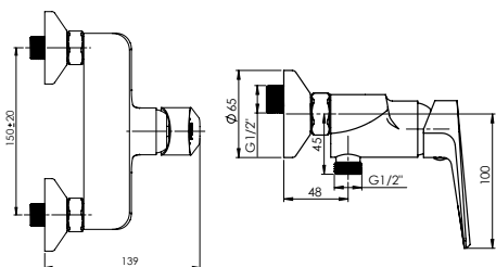
DELI-12 Sprchová batéria | D20008
