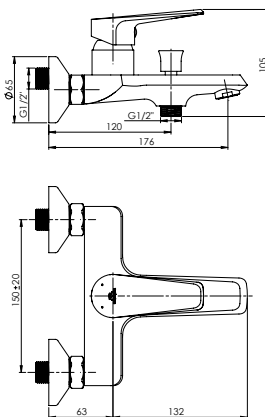
DELI-10 (K) Vaňová batéria so sprchovým setom | D10K08
