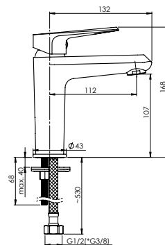
DELI-18 Umývadlová batéria | D80108
