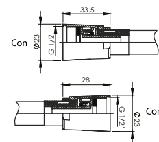
150 cm, PVC (360°) Con/Con, Black PVC sprchová hadica, čierna, 150 cm, Con/Con | 600064B
