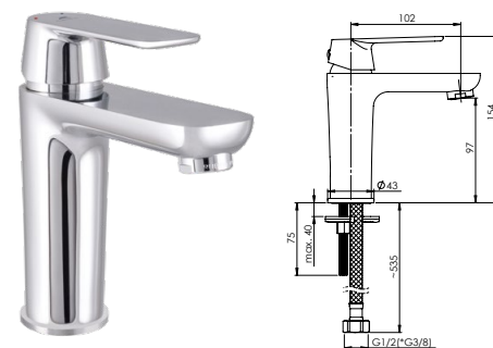
ELMA-18 Umývadlová batéria | EL80108
