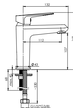
DELI-18 Praustuvės maišytuvas | D80008
