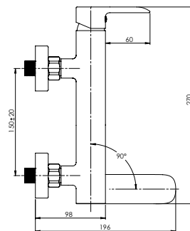
ULTRA-10 (SW) (K) Vonios / dušo maišytuvas su dušo rinkiniu | U1KP08
